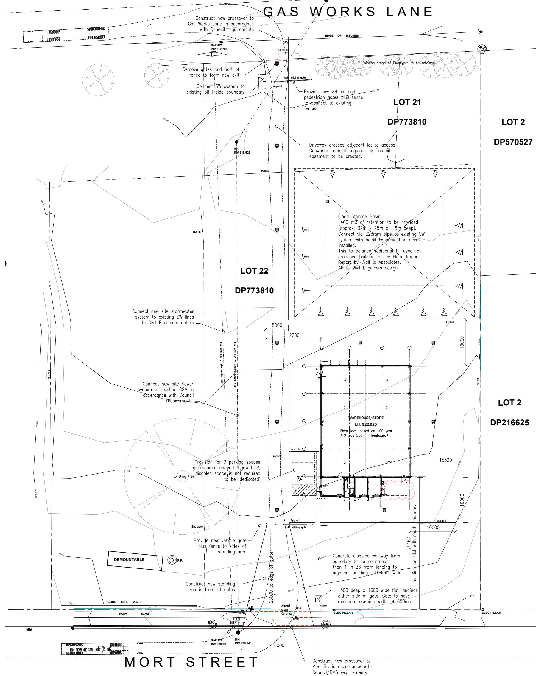
SITE PLAN 1:500
